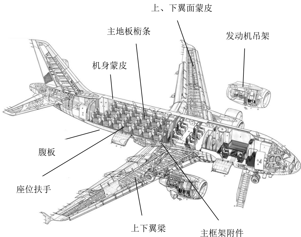
飞机用铝合金示意图
